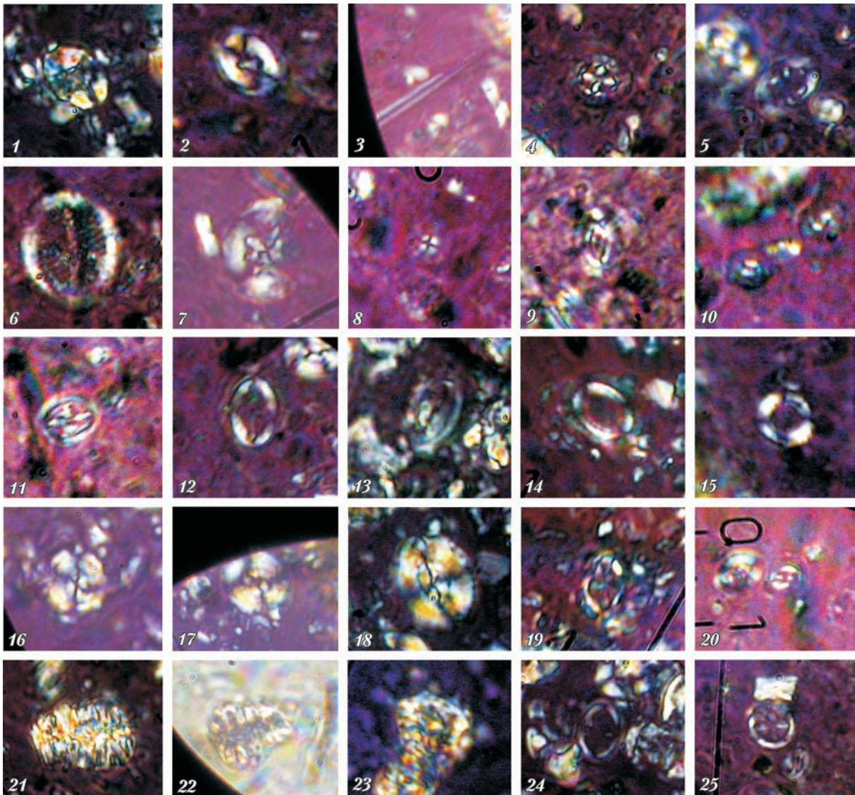
Рис. 2. Вапняковий нанопланктон з крейдових відкладів Фороського виступу Кримського континентального схилу, зображення в схрещених ніколах 90°, зб. 1575 (масштабність знімків не витримувалась із змінами розмірів у програмі Adobe Photoshop): 1 – Eiffellithus turiseiffelii (Deflandre) Reinhardt, зразок 5862/6, 62-й рейс НДС “Професор Водяницький”; 2 – Eiffellithus sp., зразок 5806/5, 62-й рейс НДС “Професор Водяницький”; 3 – Lithraphidites carniolensis Deflandre, зразок 5806/5, 62-й рейс НДС “Професор Водяницький”; 4 – Prediscosphaera sp., зразок 5806/5, 62-й рейс НДС “Професор Водяницький”; 5 – Tegumentum stradneri Thierstein, зразок 3-27/20, 27-й рейс НДС “Володимир Паршин”; 6 – Cretarhabdus aff. striatus (Stradner) Black, зразок 5806/5, 62-й рейс НДС “Професор Водяницький”; 7 – Retecapsa angustiforata Black, зразок 3-27/20, 27-й рейс НДС “Володимир Паршин”; 8 – Discorhabdus ignotus (Gorka) Perch-Nielsen, зразок 5800/2, 61-й рейс НДС “Професор Водяницький”; 9 – Biscutum constans (Gorka) Black, зразок 5746/1, 59-й рейс НДС “Професор Водяницький”; 10 – Biscutum sp., зразок 5806/5, 62-й рейс НДС “Професор Водяницький”; 11 – Staurolithites sp., зразок 3-27/20, 27-й рейс НДС “Володимир Паршин”; 12 – ? Staurolithites aff. glabra (Jeremiah) Burnett, зразок 3-27/20, 27-й рейс НДС “Володимир Паршин”; 13 – Tranolithus sp., зразок 3-27/10, 27-й рейс НДС “Володимир Паршин”; 14 – Cribrosphaerella ehrenbergii (Arkhangelsky) Deflandre, зразок 5862/6, 62-й рейс НДС “Професор Водяницький”; 15 – ? Diazomatolithus cf. D. lehmanii Noël, зразок 3-27/20, 27-й рейс НДС “Володимир Паршин”; 16 – Watznaueria barnesae (Black) Perch-Nielsen, зразок 3-27/10, 27-й рейс НДС “Володимир Паршин”; 17 – Watznaueria fossacincta (Black) Worn, зразок 3-27/10, 27-й рейс НДС “Володимир Паршин”; 18 – Watznaueria manivittiae Bukry, зразок 5862/6, 62-й рейс НДС “Професор Водяницький”; 19 – Helicolithus aff. compactus (Bukry) Varol and Girgis, зразок 3-27/10, 27-й рейс НДС “Володимир Паршин”; 20 – Crucibiscutum hayi (Black) Jakubowski, зразок 5806/5, 62-й рейс НДС “Професор Водяницький”; 21 – Nannoconus aff. kamptneri Brönnimann kamptneri , зразок 5629/4, 57-й рейс НДС “Професор Водяницький”; 22 – Nannoconus kamptneri Brönnimann minor Bralower, зразок 5629/4, 57-й рейс НДС “Професор Водяницький”; 23 – Nannoconus aff. aquitanicus Deres and Acheritequy, зразок 5862/8, 62-й рейс НДС “Професор Водяницький”; 24 – Placozygus sp., зразок 280/5, 7-й рейс НДС “Київ”; 25 – Stoverius achylosus (Stover) Perch-Nielsen, зразок 3-27/20, 27-й рейс НДС “Володимир Паршин”
