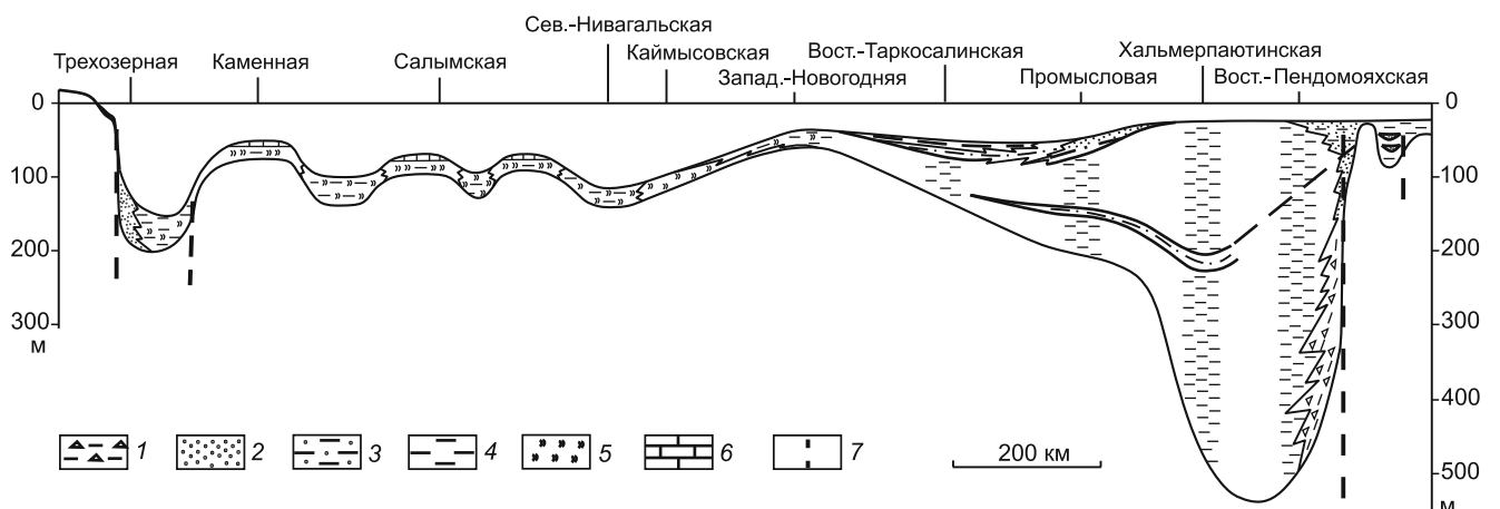
Рис. 3. Структурно-фациальный профиль Западно-Сибирского бассейна в титоне-раннем берриасе: 1 — осадочные брекчии; 2 — песчаники; 3 — алевролиты; 4 — аргиллиты; 5 — кремнистые породы; 6 — известняки; 7 — конседиментационные разломы
