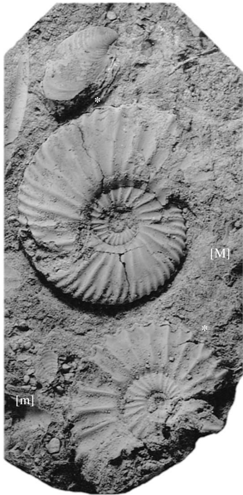
Рис. 1. Макро- и микроконх Riasanites rjasanensis (Nikitin) morpha \beta в одном куске фосфоритового песчаника, экз. № 3990/294. Рязанская обл., берег р. Оки ниже д. Никитино; рязанский ярус, зона Riasanites rjasanensis , фаунистический комплекс с Surites spasskensis . Звездочкой отмечено начало жилой камеры ( \times 0.9 ).
